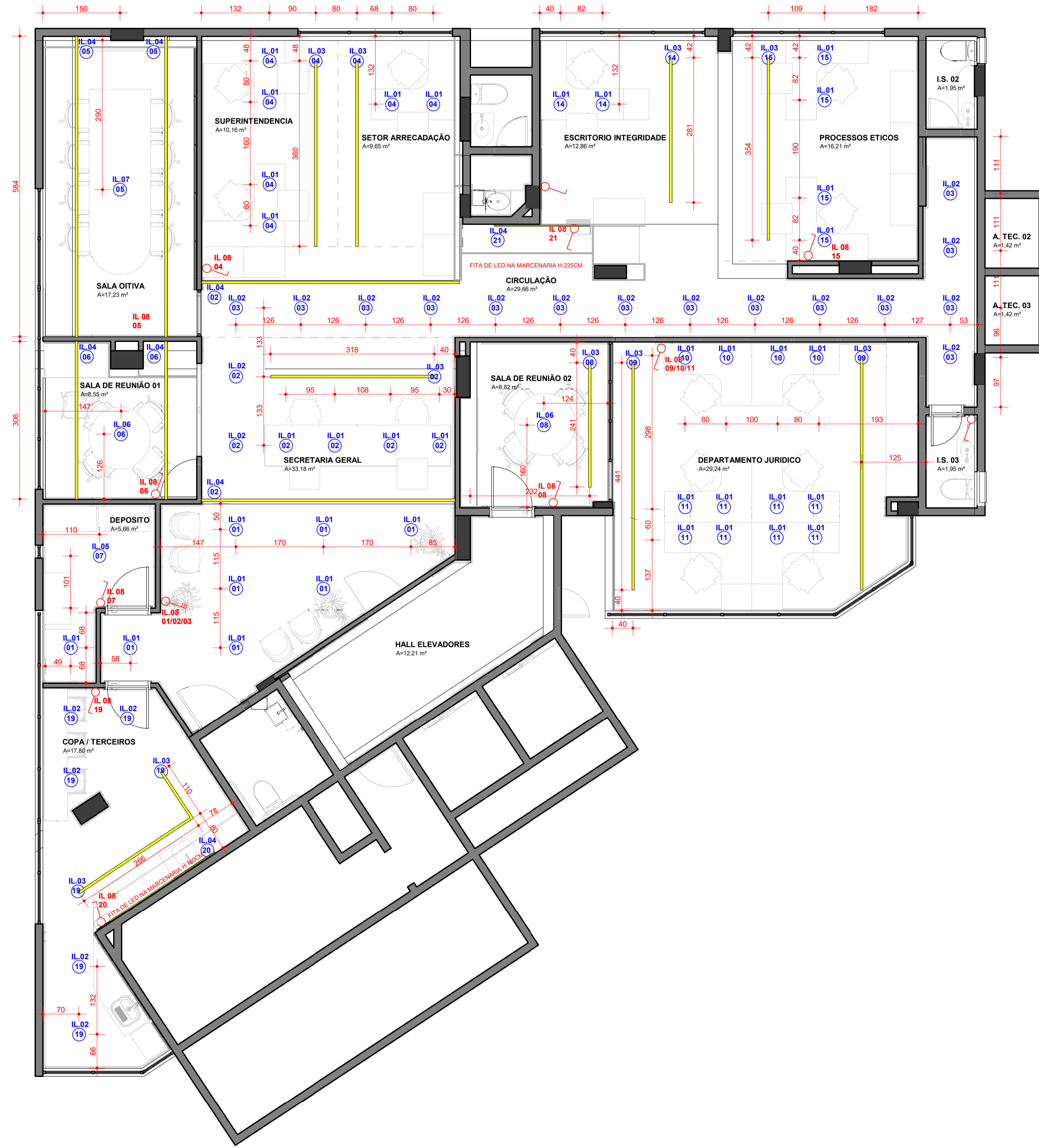
01 PLANTA BAIXA LUMINOTECNICO - 5º PAVIMENTO ESCALA 1:50
